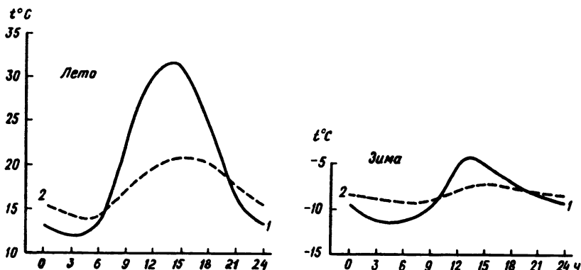
Рис. 5.2. Средний суточный ход температуры на поверхности почвы (1) и в воздухе на высоте 2 м (2) летом и зимой. Москва (МГУ)
