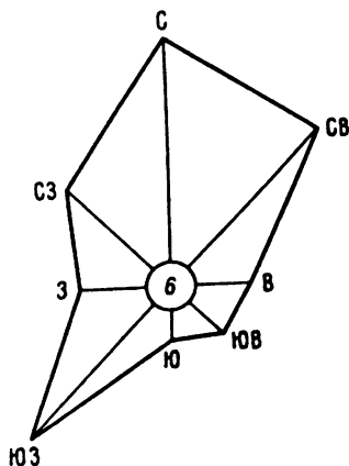
Рис. 2.6. Роза ветров
