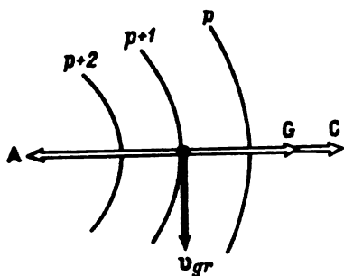
Рис. 4.16. Градиентный ветер в антициклоне. Условные обозначения см. на рис. 4.15
