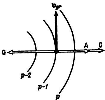
Рис. 4.15. Градиентный ветер в циклоне: G — сила барического градиента, A — отклоняющая сила вращения Земли, C — центробежная сила, v — скорость градиентного ветра
