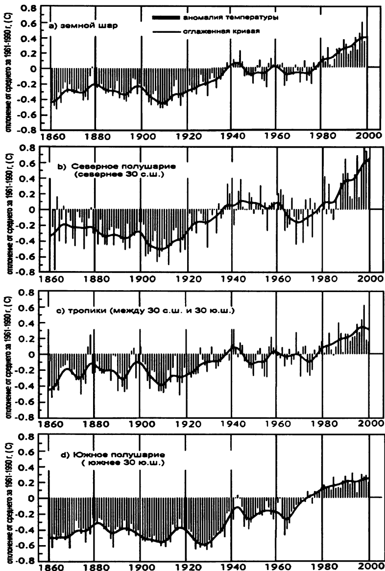
Рис. 10.4. Временной ход среднегодовых аномалий температуры воздуха ( ^{\circ}\text{C} ) у поверхности Земли с 1861 по 2000 г. (в отклонениях от нормы за 1961—1990 г.): a — для всего Земного шара; b — для Северного полушария к северу от 30^{\circ} с.ш.; c — для тропиков между 30^{\circ} с.ш. — 30^{\circ} ю.ш.; d — для Южного полушария к югу от 30^{\circ} ю.ш. Сглаженная кривая — результат скользящего осреднения с характерным временем 10 лет в указанных выше зонах (Climatic Research Unit, University of East Anglia and Hadley Center, The Met Office)
