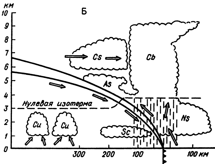
Рис. 4.23. Теплый (А) и холодный (Б) фронты (вертикальный разрез)
