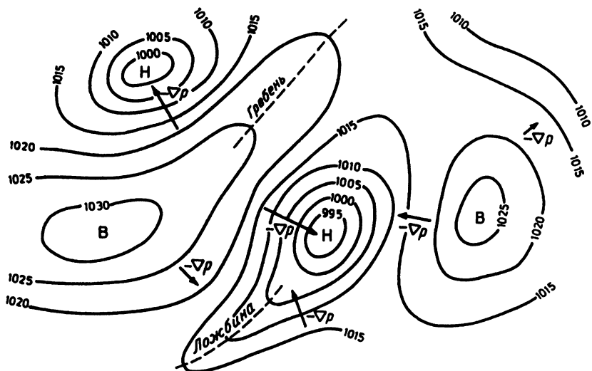
Рис. 4.1. Изобары на уровне моря (гПа) и горизонтальный барический градиент: H — циклон, B — антициклон. Стрелками обозначен горизонтальный барический градиент в шести точках барического поля
