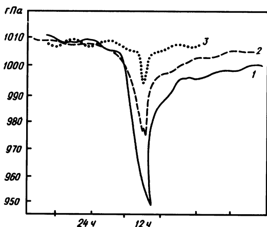
Рис. 7.10. Изменение давления на о. Мадагаскар в феврале—марте 1959 г. при прохождении тропических циклонов: 1 — жестокого, 2 — умеренного, 3 — слабого
