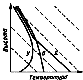
Рис. 5.16. Изменение атмосферной стратификации над сушей в суточном ходе: У — на восходе Солнца, Д — около полудня, В — вечером
