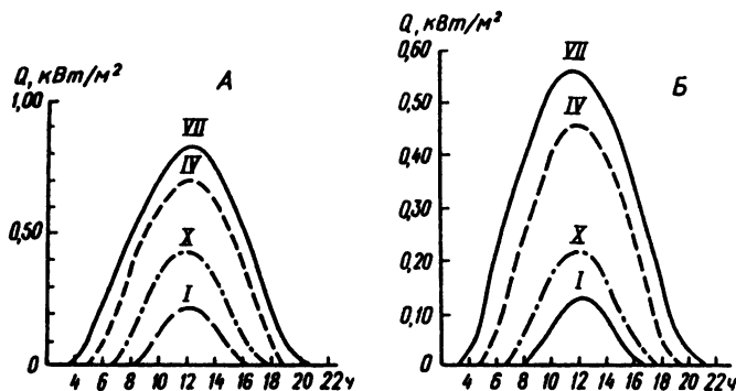
Рис. 3.8. Дневной ход суммарной солнечной радиации в Москве (данные обсерватории МГУ) в январе, апреле, июле и октябре при ясном небе (а) и при средних условиях облачности (б)
