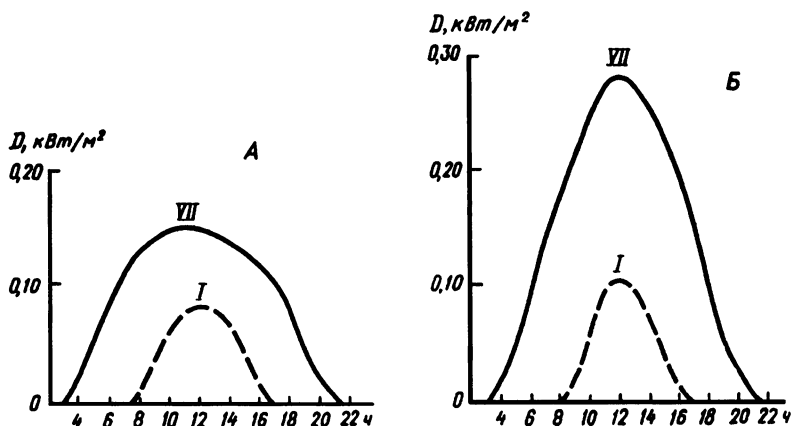
Рис. 3.7. Дневной ход рассеянной солнечной радиации в Москве (данные обсерватории МГУ) в январе и июле при ясном небе (а) и при средних условиях облачности (б)
