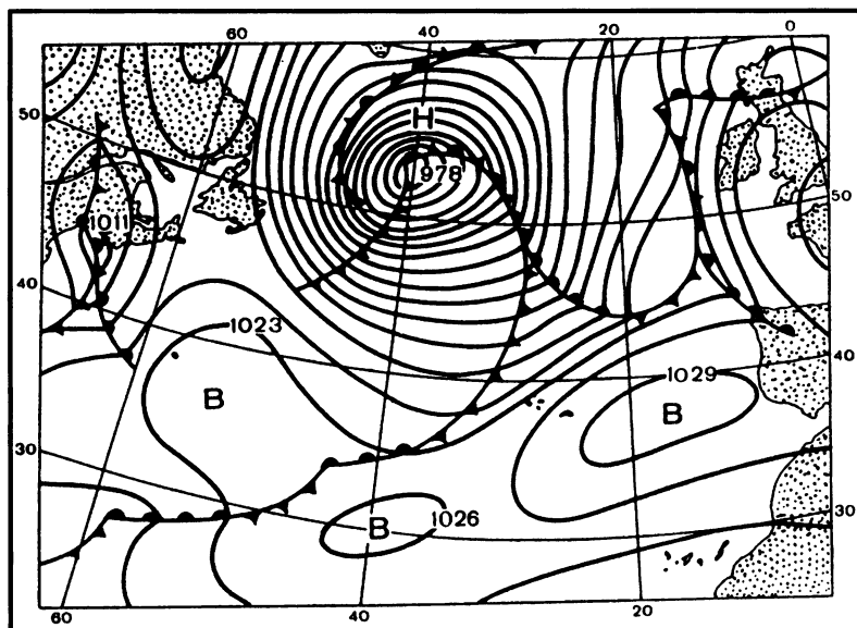
Рис. 7.18. Центральный циклон и субтропический антициклон на синоптической карте (карта упрощена, оставлены только изобары и фронты)
