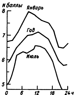
Рис. 6.10. Суточный ход облачности в Потсдаме
