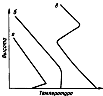
Рис. 5.17. Типы распределения температуры с высотой: a — приземная инверсия, b — приземная изотермия, v — инверсия в свободной атмосфере
