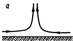
Рис. 2.10. Связь сходимости (а) и расходимости (б) с вертикальными движениями (вертикальный разрез)
