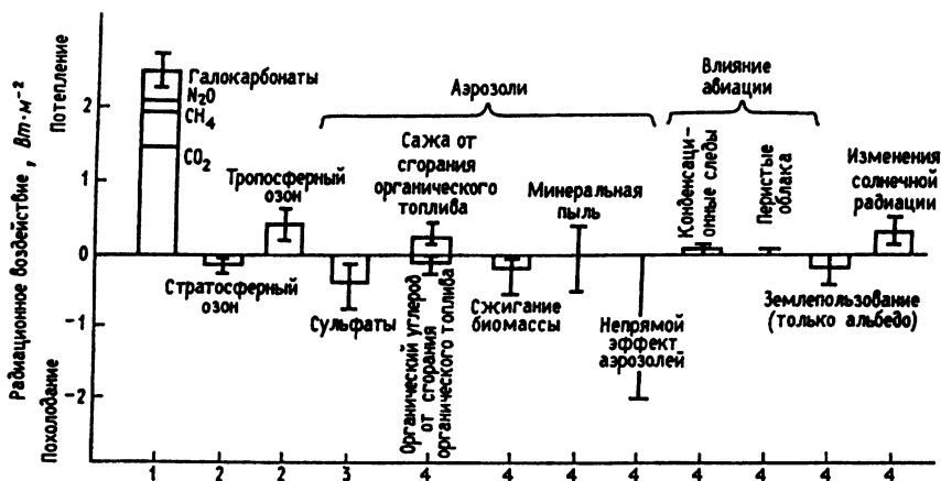
Рис. 10.5. Осредненное по земному шару радиационное воздействие на климатическую систему внешних факторов в 2000 г. по отношению к 1750 г. Столбики — оценки вклада рассматриваемых факторов; вертикальная линия на вершине столбика указывает диапазон оценок с учетом разброса опубликованных значений и понимания физики явления; вертикальная черта без столбика означает воздействие, для которого лучшей оценки получить нельзя из-за больших неопределенностей. Цифрами под рисунком указано качество оценки каждого фактора по следующей шкале: 1 — высокое; 2 — среднее; 3 — низкое; 4 — очень низкое (по: Израэль Ю.А., Груза Г.В., Катцов В.М., Мелешко В.П. Метеорология и гидрология. 2001. № 5. С. 5—21)
