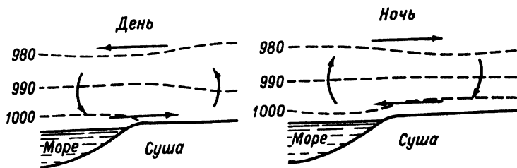
Рис. 7.22. Схема бризов
