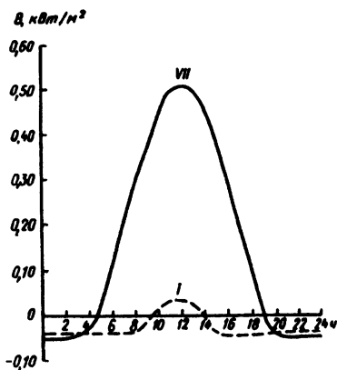
Рис. 3.10. Суточный ход радиационного баланса в Москве (МГУ) в январе и июле
