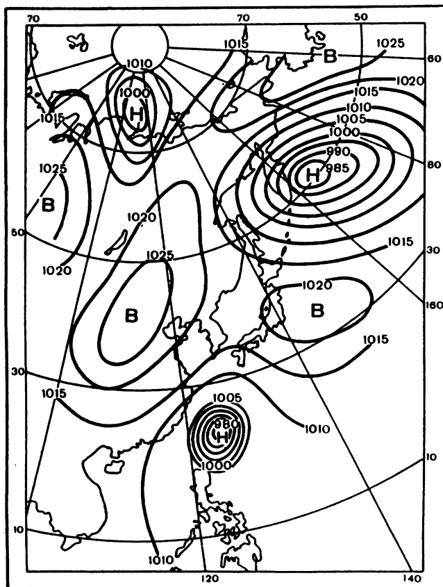
Рис. 7.9. Тайфун и внетропический циклон на карте давления
