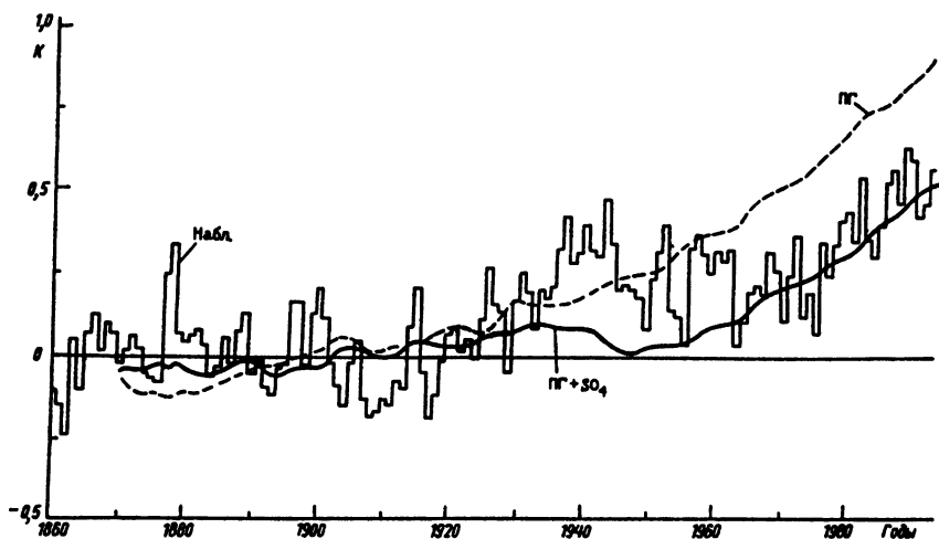
Рис. 10.6. Временной ход наблюдаемых среднегодовых аномалий температуры («набл») с 1860 по 1987 г. (в отклонениях от нормы за 1951—1980 гг.), результаты интегрирования Глобальной климатической модели (атмосфера—океан) с учетом радиационного воздействия от реального изменения концентрации парниковых газов («ПГ») и результаты интегрирования этой же модели с учетом радиационного воздействия парниковых газов и антропогенного сернокислотного аэрозоля («ПГ+SO 4 ») (Mitchell J.F.B., Johns T.J., Gregory J.M., Tett S.B.F. Nature. 1995. Vol. 376. P. 501—504)
