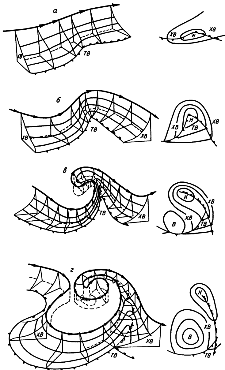
Рис. 7.13. Схема развития фронтального циклона: пространственное положение фронта у Земли, на 850, 700, 500 гПа и струйное течение на 300 гПа (слева), положение фронтов и изобары у Земли (справа); а — волна, б — молодой циклон, в — окклюдированный циклон — максимальное развитие, г — окклюдированный циклон — заключительная стадия
