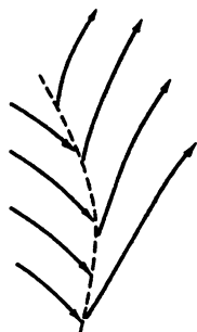
Рис. 2.9. Односторонняя линия сходимости
