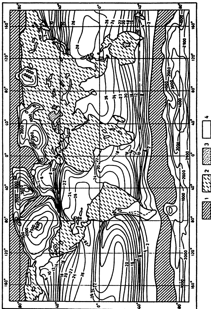
Рис. 10.2. Реконструкция климата поверхности Земли в ав- густе во время максимальной стадии последнего оледенения 21 тыс. лет назад. Высота по- верхности ледниковых щитов дана в метрах, изотермы при- ведены через 2°С. Контуры ма- териков совпадают с современ- ной изобатой 85 м. Пунктиром показана граница материко- вого льда в Южной Америке. 1 — морской лед, 2 — по- верхность свободная ото льда, 3 — внутренние воды, 4 — снег и лед
