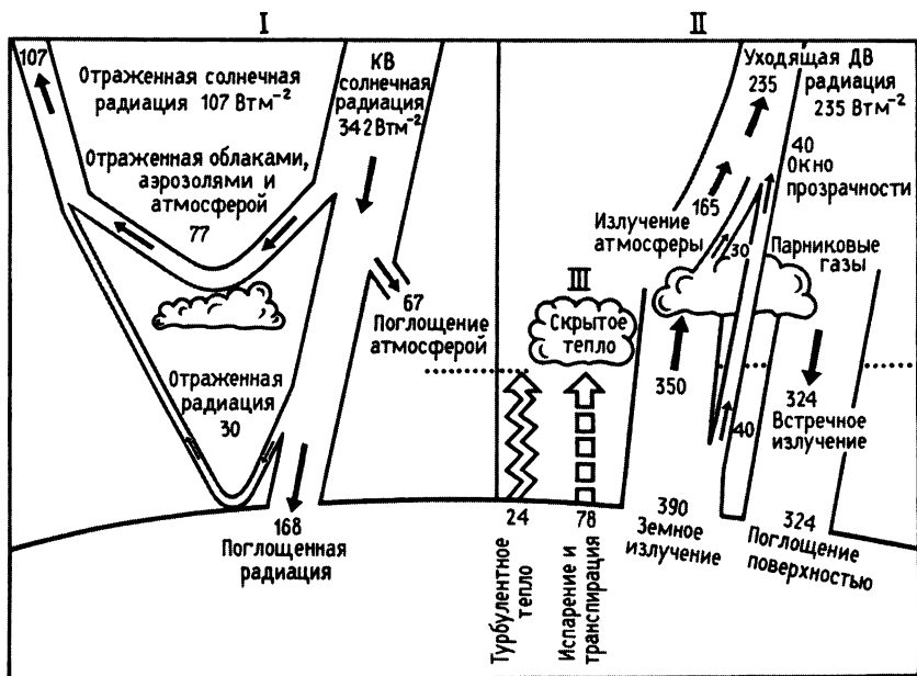
Рис. 5.21. Средний тепловой баланс Земли, атмосферы и земной поверхности: I — коротковолновая радиация, II — длинноволновая радиация, III — нерадикационный обмен
