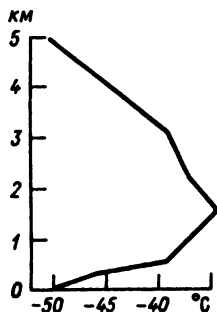
Рис. 5.18. Зимняя инверсия температуры над Якутском 2 декабря 1957 г.
