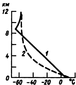
Рис. 5.14. Распределение средней температуры воздуха с высотой по фактическим данным (1) и в предположении лучистого равновесия (2)
