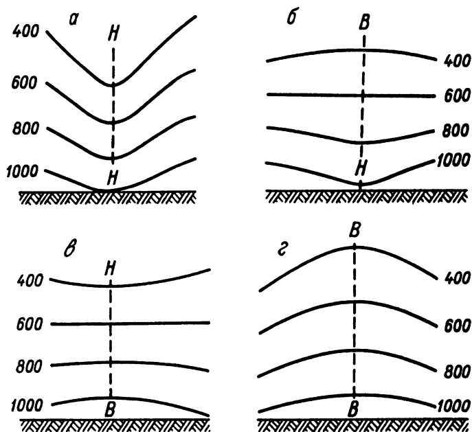
Рис. 4.10. Изобарические поверхности в вертикальном разрезе: а — высокий (холодный), б — низкий (теплый) циклон, в — низкий (холодный), г — высокий (теплый) антициклон
