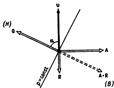
Рис. 4.18. Ветер в слое трения (равномерное прямолинейное движение воздуха при наличии силы трения): G — сила барического градиента, A — отклоняющая сила вращения Земли, R — сила трения, v — скорость ветра
