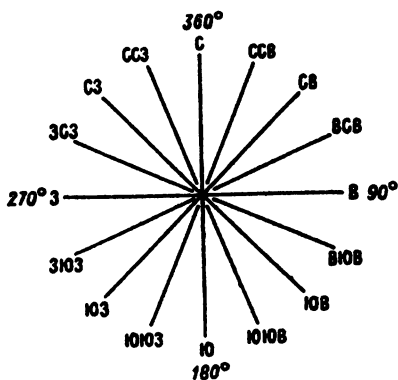
Рис. 2.5. Румбы горизонта
