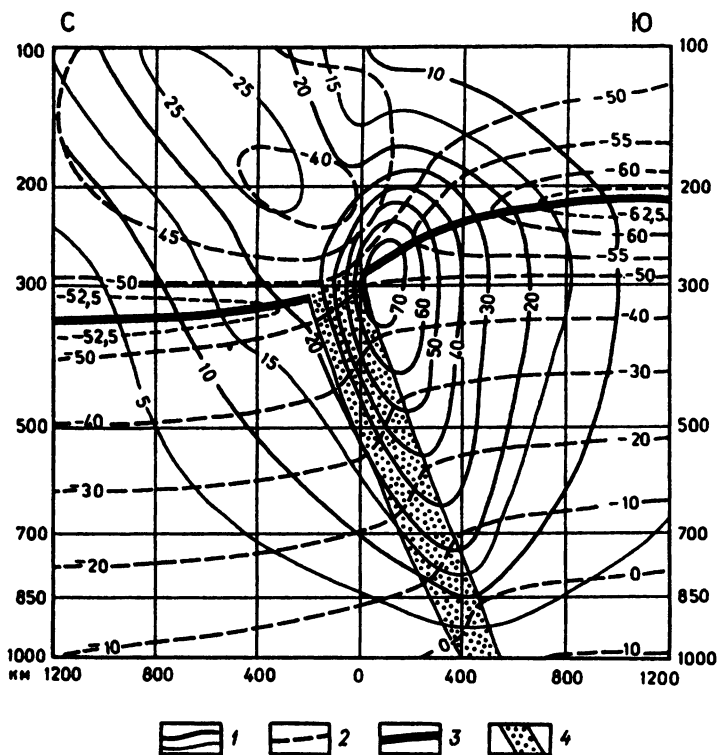
Рис. 4.25. Вертикальный разрез через струйное течение: 1 — изолинии западной составляющей скорости ветра (м/с); 2 — изотермы ( ^{\circ}\text{C} ); 3 — тропопауза в холодном и теплом воздухе; 4 — зона фронта
