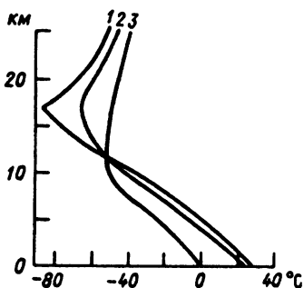
Рис. 5.12. Среднее распределение температуры воздуха с высотой на экваторе (1), под 30° с.ш. (2) и под 60° с.ш. (3)
