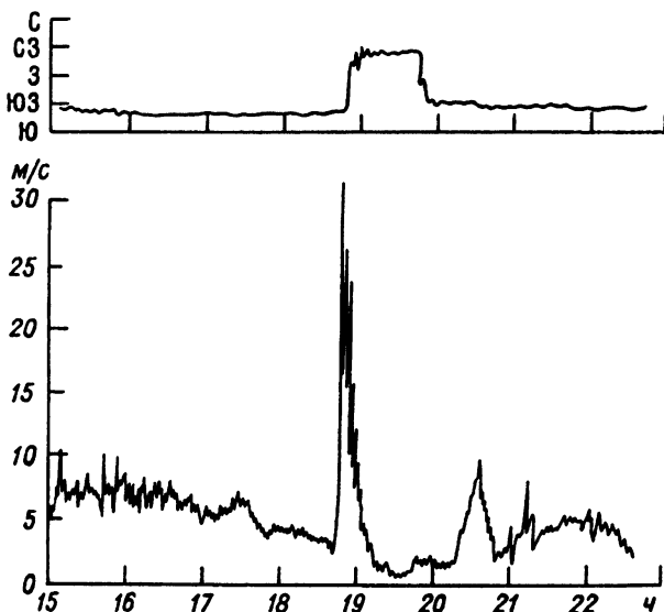
Рис. 7.25. Пример изменения скорости и направления ветра при шквале
