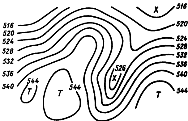
Рис. 4.5. Области тепла (Т) и холода (Х) на карте относительной топографии изобарической поверхности 500 гПа над поверхностью 1000 гПа: в областях тепла толщина атмосферного слоя между двумя поверхностями увеличена, в областях холода — уменьшена
