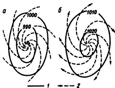
Рис. 4.19. Изобары (1) и линии тока (2) в нижних слоях циклона (а) и антициклона (б)
