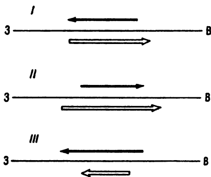
Рис. 4.22. Типы распределения ветра по обе стороны фронта в горизонтальной плоскости, соответствующие трем типам распределения давления (см. рис. 4.21)
