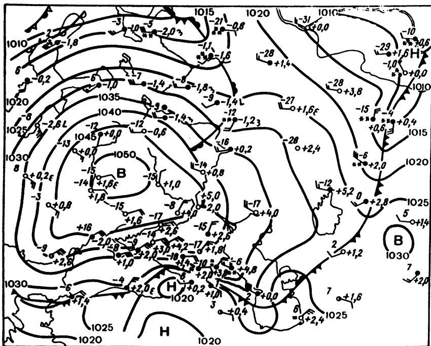
Рис. 7.19. Антициклон на синоптической карте
