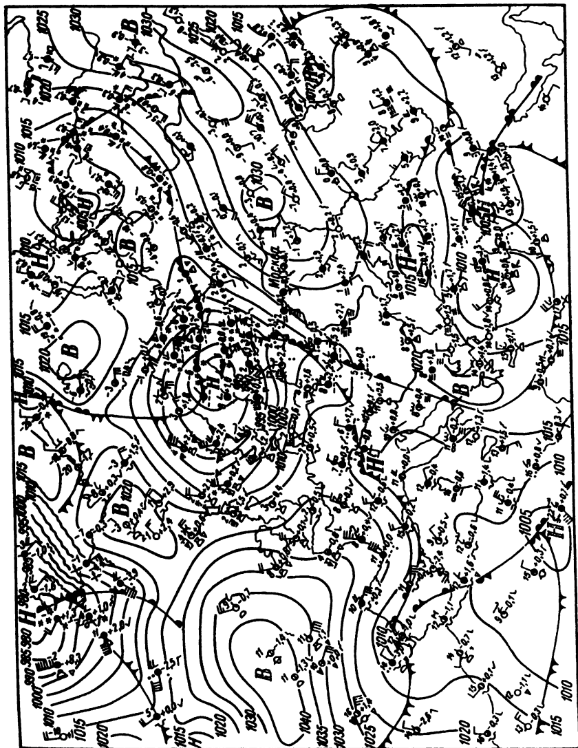
Рис. 7.28. Синоптическая карта
