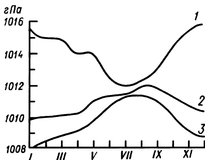
Рис. 7.1. Годовой ход среднего давления воздуха в Северном полушарии (1), в экваториальной зоне между 2,5° ю.ш. (2) и в Южном полушарии (3)
