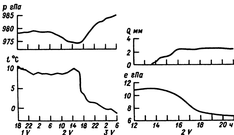
Рис. 4.24. Изменение метеорологических величин в случае прохождения холодного фронта в Москве
