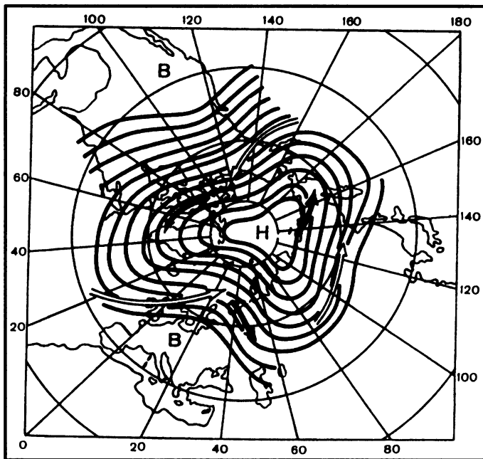
Рис. 7.20. Пример зонального типа циркуляции на карте абсолютной топографии поверхности 500 гПа
