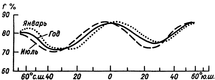
Рис. 6.7. Распределение зональной относительной влажности в зависимости от географической широты
