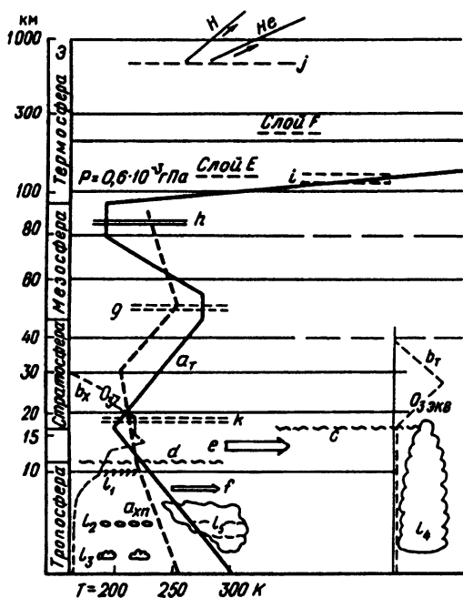
Рис. 2.1. Строение атмосферы: a — распределение температуры ( a_T — в тропиках, a_{х.п.} — в холодной полярной зоне); b_T и b_{п.} — распределение озона в тропической и полярной зонах; c — тропопауза тропическая; d — тропопауза полярная; e — струйное течение субтропическое; f — струйное течение полярное; g — стратопоауза; h — мезопоауза; i — турбопауза; j — уровень диссипации — ускользания атомов H и He; k — слой стратосферного аэрозоля; l_1, l_2, l_3, l_4, l_5 — тропосферные облака: перистые, высококучевые, кучевые, кучево-дождевые, фронтальные; э — экзосфера
