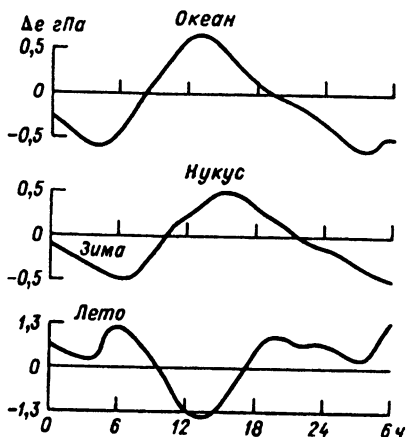
Рис. 6.3. Суточный ход давления водяного пара в тропическом океане и пустыне (г. Нукус) зимой и летом: \Delta e — отклонение от средних суточных значений
