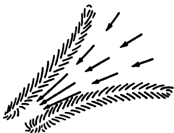
Рис. 2.11. Орографическое усиление ветра
