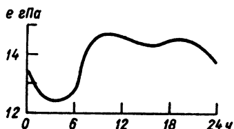
Рис. 6.4. Суточный ход давления водяного пара в Иркутске в июле
