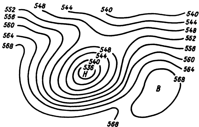
Рис. 4.3. Циклон ( H ) и антициклон ( B ) на карте абсолютной топографии изобарической поверхности 500 гПа: цифры — высоты в геопотенциальных декаметрах; в циклоне изобарическая поверхность лежит ближе к уровню моря, чем в антициклоне
