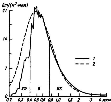
Рис. 3.1. Распределение лучистой энергии в спектре солнечной радиации до поступления в атмосферу (1) и в спектре абсолютно черного тела при температуре 6000°C (2). Области спектра: УФ — ультрафиолетовая; В — видимая; ИК — инфракрасная; спектральная плотность радиации дана в Вт/м 2 для интервала длин волн 0,01 мкм
