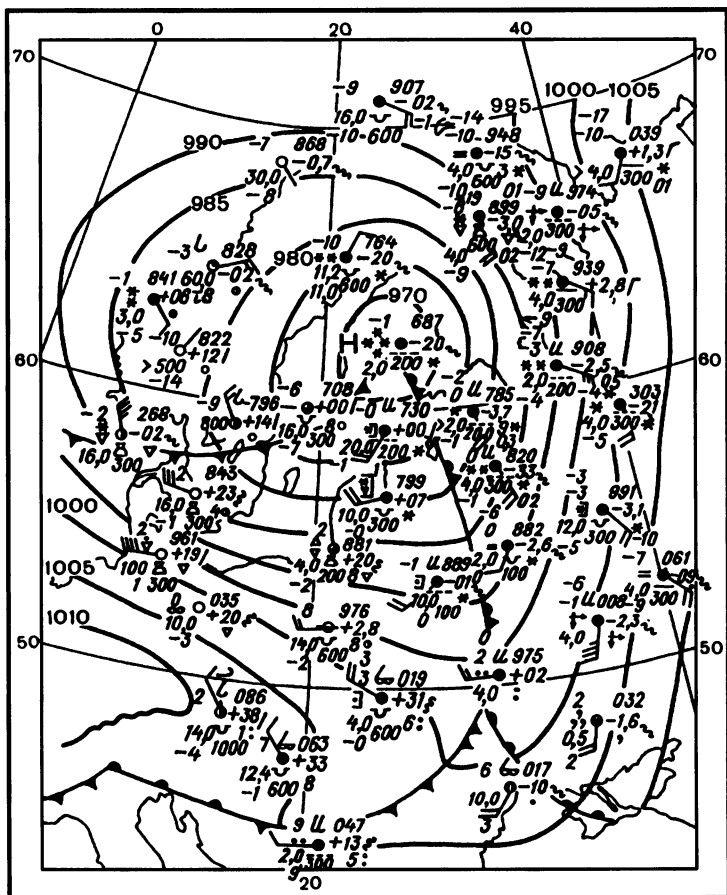
Рис. 7.12. Внетропический циклон на синоптической карте
