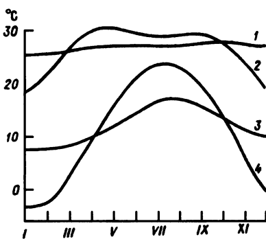
Рис. 5.10. Некоторые типы годового хода температуры воздуха: 1 — экваториальный (Джакарта), 2 — тропический в области муссонов (Калькутта), 3 — морской в умеренном поясе (Силли, Шотландия), 4 — континентальный в умеренном поясе (Чикаго)
