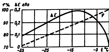
Рис. 6.2. Разность давления насыщения над водой и льдом и относительная влажность при насыщении надо льдом в зависимости от температуры
