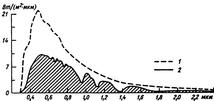
Рис. 3.3. Распределение энергии в спектре солнечной радиации на границе атмосферы (1) и у земной поверхности (2) при высоте солнца 35^\circ : спектральная плотность радиации дана в \text{Вт}/\text{м}^2 для интервала длин волн 0,01 \text{ мкм}
