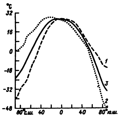
Рис. 5.11. Зависимость средней температуры воздуха у земной поверхности от географической широты: 1 — январь, 2 — июль, 3 — год
