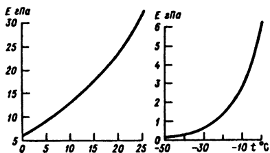
Рис. 6.1. Давление насыщенного водяного пара в зависимости от температуры
