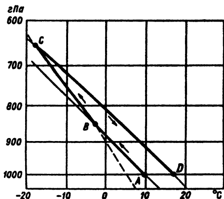
Рис. 2.4. Псевдоадиабатический процесс в координатах температура—давление: от точки A до точки B температура воздуха падает по сухоадиабатическому закону, от точки B до точки C — по влажноадиабатическому закону, от точки C до точки D — растет по сухоадиабатическому закону
