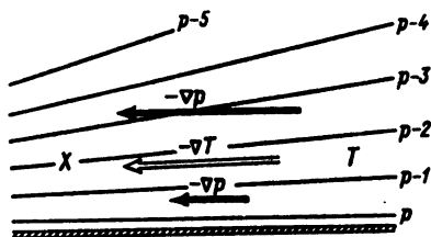
Рис. 4.7. Связь между горизонтальными градиентами температуры и давления
