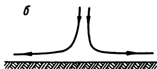
Рис. 2.10. Связь сходимости (а) и расходимости (б) с вертикальными движениями (вертикальный разрез)
