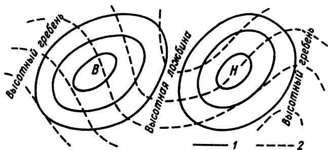
Рис. 4.9. Изобары в циклоне ( H ) и антициклоне ( B ) на уровне моря (1) и на более высоком уровне (2)
