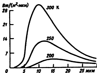
Рис. 3.9. Излучение абсолютно черного тела при температурах 200, 250 и 300 К
