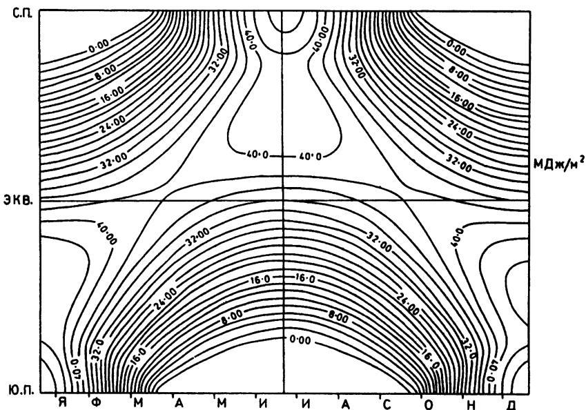
Рис. 3.12. Изоплеты суточного притока солнечной радиации на горизонтальную поверхность на верхней границе атмосферы (Мдж/м 2 ) в зависимости от широты и времени года
