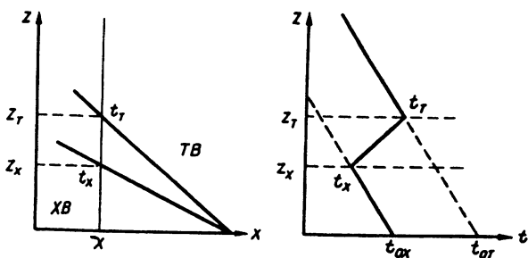
Рис. 5.20. Фронтальная зона и образование фронтальной инверсии: Z_X — верхняя граница холодной воздушной массы в пункте X ; Z_T — нижняя граница теплой воздушной массы в пункте X ; Z_T - Z_X — толщина фронтальной зоны в пункте X ; t_X — температура на верхней границе холодной воздушной массы в пункте X ; t_T — температура на нижней границе теплой воздушной массы в пункте X ; t_T - t_X — значение инверсии температуры во фронтальной зоне
