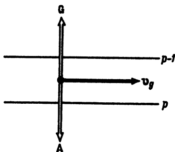
Рис. 4.14. Геострофический ветер: G — сила барического градиента, A — отклоняющая сила вращения Земли, v_g — скорость ветра
