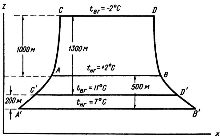
Рис. 5.19. Образование инверсии сжатия
