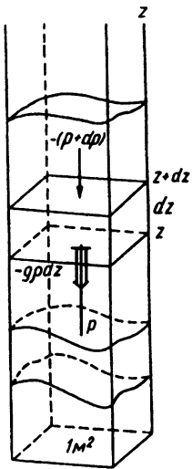
Рис. 2.2. Силы, действующие на элементарный объем воздуха по вертикали
