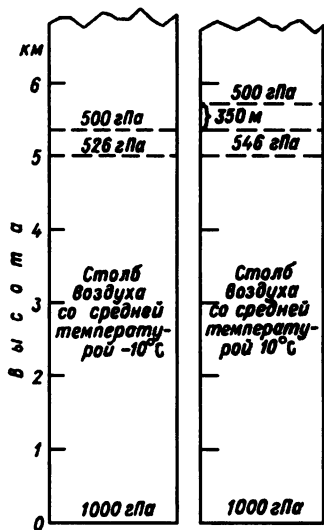
Рис. 2.3. Убывание атмосферного давления с высотой в зависимости от температуры воздушного столба: при одинаковом давлении внизу давление 500 гПа в теплом столбе наблюдается на 350 м выше, чем в холодном
