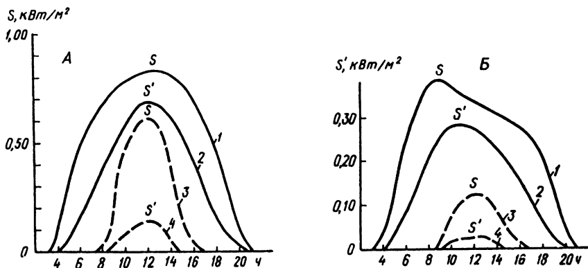
Рис. 3.5. Дневной ход прямой солнечной радиации в Москве в январе и июле при ясном небе (а) и при средних условиях облачности (б): 1 — на поверхность, перпендикулярную к лучам в июле, 2 — на горизонтальную поверхность в июле, 3 — на перпендикулярную поверхность в январе, 4 — на горизонтальную поверхность в январе
