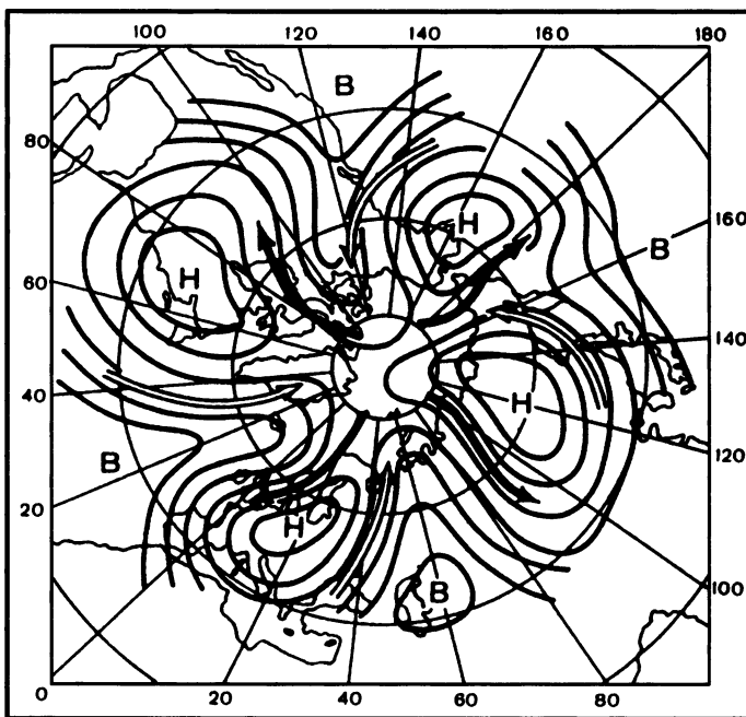
Рис. 7.21. Пример меридионального типа циркуляции на карте абсолютной топографии поверхности 500 гПа
