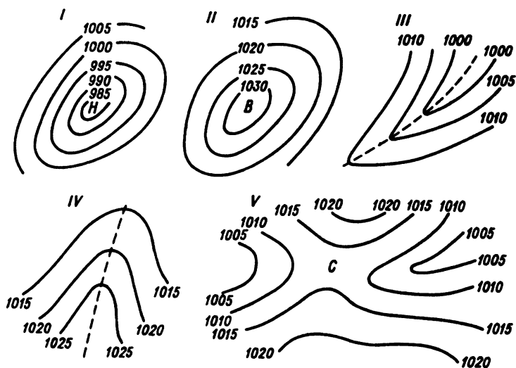
Рис. 4.8. Изобары на уровне моря в различных типах барических систем: I — циклон; II — антициклон; III — ложбина; IV — гребень; V — седловина
