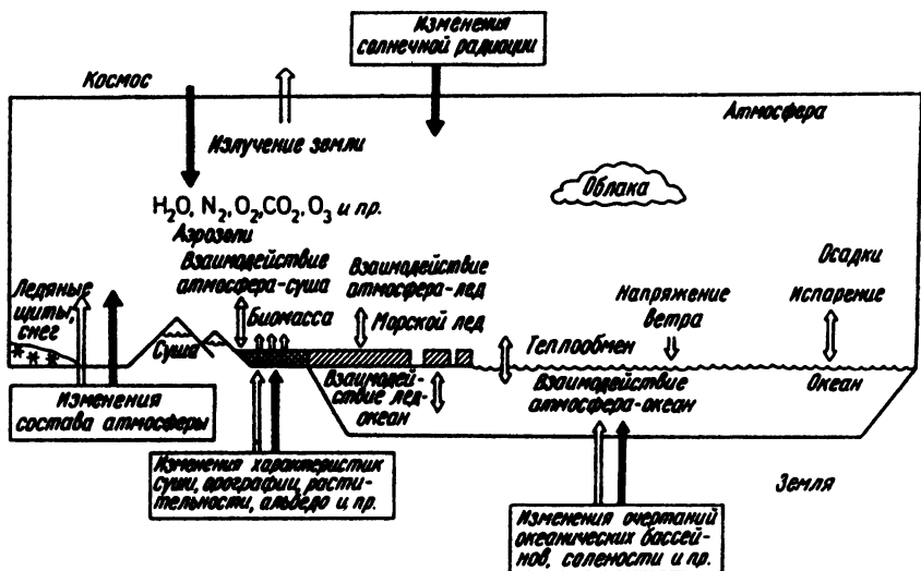
Рис. 8.1. Компоненты климатической системы атмосфера—океан—поверхность снега, льда и суши — биомасса (схема); зачерненные стрелки — внешние процессы, светлые стрелки — внутренние процессы, приводящие к изменениям климата
